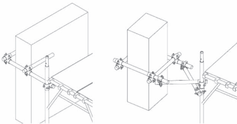
Tipologie di ancoraggio a cravatta (Fonte Marcegaglia SpA)
