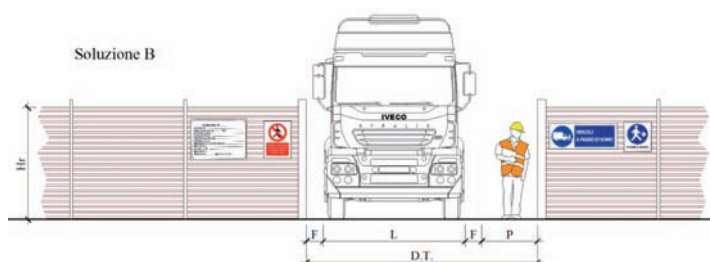
Soluzione B. Unico accesso al cantiere: ingresso veicolare e pedonale
