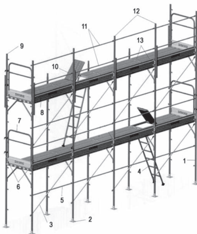
Elementi del ponteggio: 1) telaio; 2) basetta; 3) diagonale di facciata; 4) scala; 5) e 11) correnti; 6) ganci di sicurezza; 7) parapetto di testata; 8) tavola fermapiede; 9) e 12) montanti di sommità; 10) tavolato metallico con botola; 13) tavolato metallico (Fonte SOCOME SpA)
