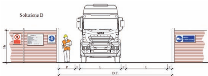
Soluzione D. Come la soluzione B ma con accesso veicolare doppio per l'entrata e l'uscita dei mezzi di cantiere
