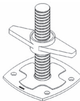
Tipologie di basette inclinabili e regolabili (Fonte Ponteggi Eurotempo SpA)
