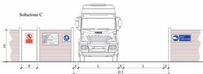
Soluzione C. Come la soluzione A ma con accesso veicolare doppio per l'entrata e l'uscita dei mezzi di cantiere
