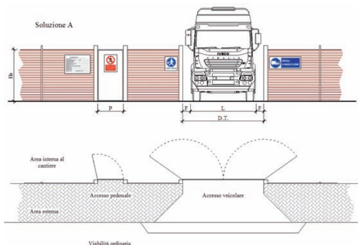
Soluzione A. Accesso pedonale ed unico ingresso veicolare
